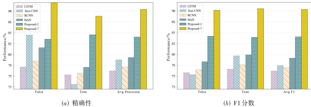
图 7 PHEME→Weibo 检测性能对比
