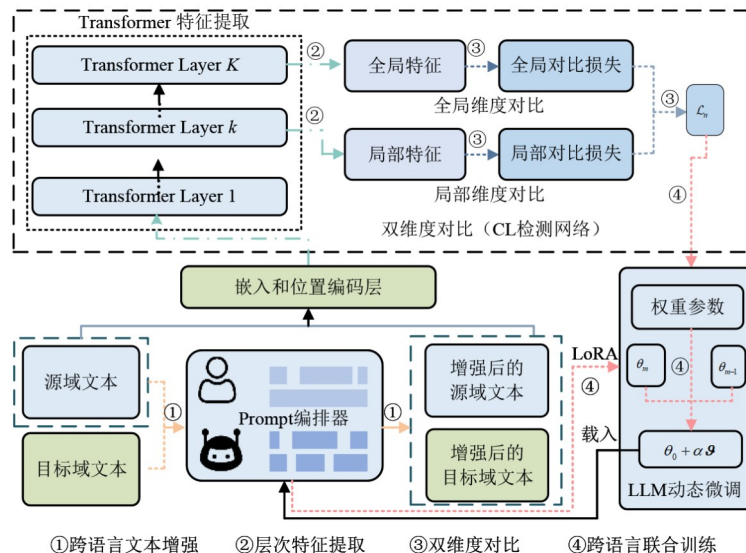
图 1 LLM 辅助的双维度跨语言检测框架
