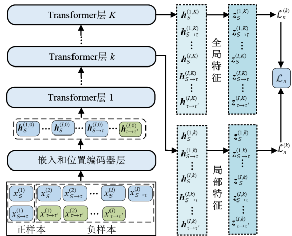
图4 双维度对比架构
