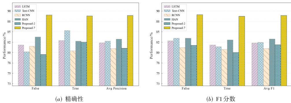
图 6 Weibo→PHEME 检测性能对比
